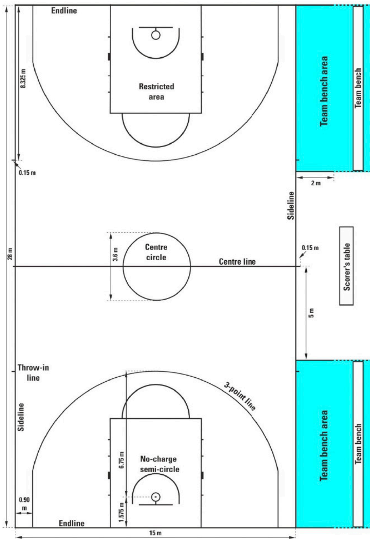
ภาพที่ 1 สนามแข่งขัน: Full size court
